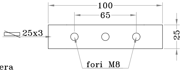
Particolare traversi portamorsettiera
