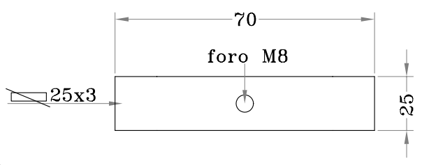
Particolare traversi portamorsettiera
